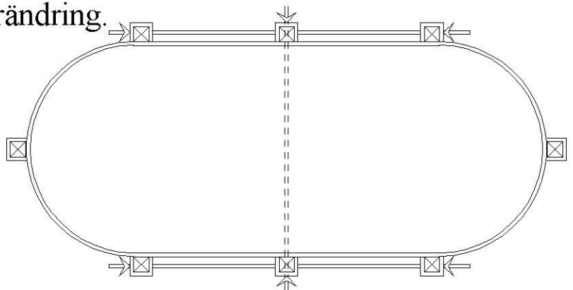
Tvårsnitt av oval pelareform - de raka delarna är genombultrade
